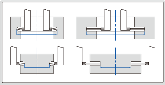
测量内凹槽和外凹槽
